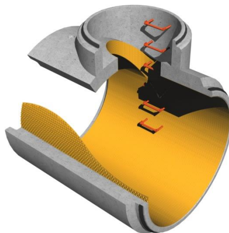
Tubo prefabbricato d'ispezione con rivestimento in PE 'liner'
