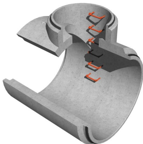
Tubo prefabbricato d'ispezione
